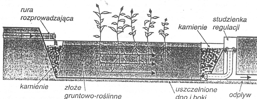
Filtr gruntowo-wodny o przepływie poziomym
