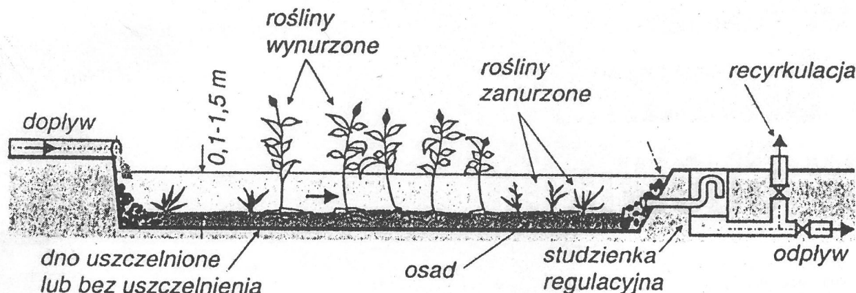
Zbiornik z zakorzenioną roślinnością
